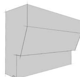
Profili per sottodavanzali StoDeco 03899-009 Spessore 120 mm Tipo PV-1000-230 Altezza 200 mm FBG-030 Lunghezza 2400 mm
