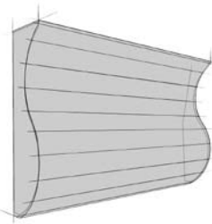
Supporti per davanzali StoDeco 03937-002 Spessore 80 mm Tipo PV-1000-655 Altezza 300 mm Lunghezza 180 mm
