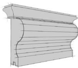
Supporti per davanzali StoDeco 03937-002 Spessore 40 mm Tipo PV-1000-652 Altezza 100 mm Lunghezza 180 mm
