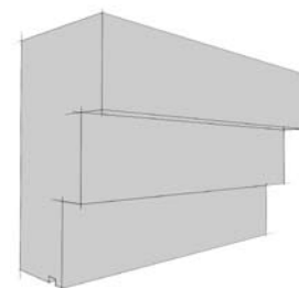
Profili per sottodavanzali StoDeco 03899-009 Spessore 120 mm Tipo PV-1000-227 Altezza 200 mm FBG-027 Lunghezza 2400 mm
